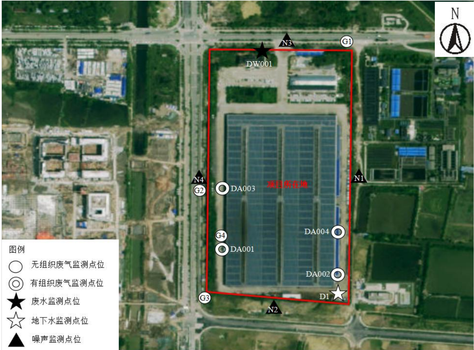
附图 8 项目验收监测点位图
