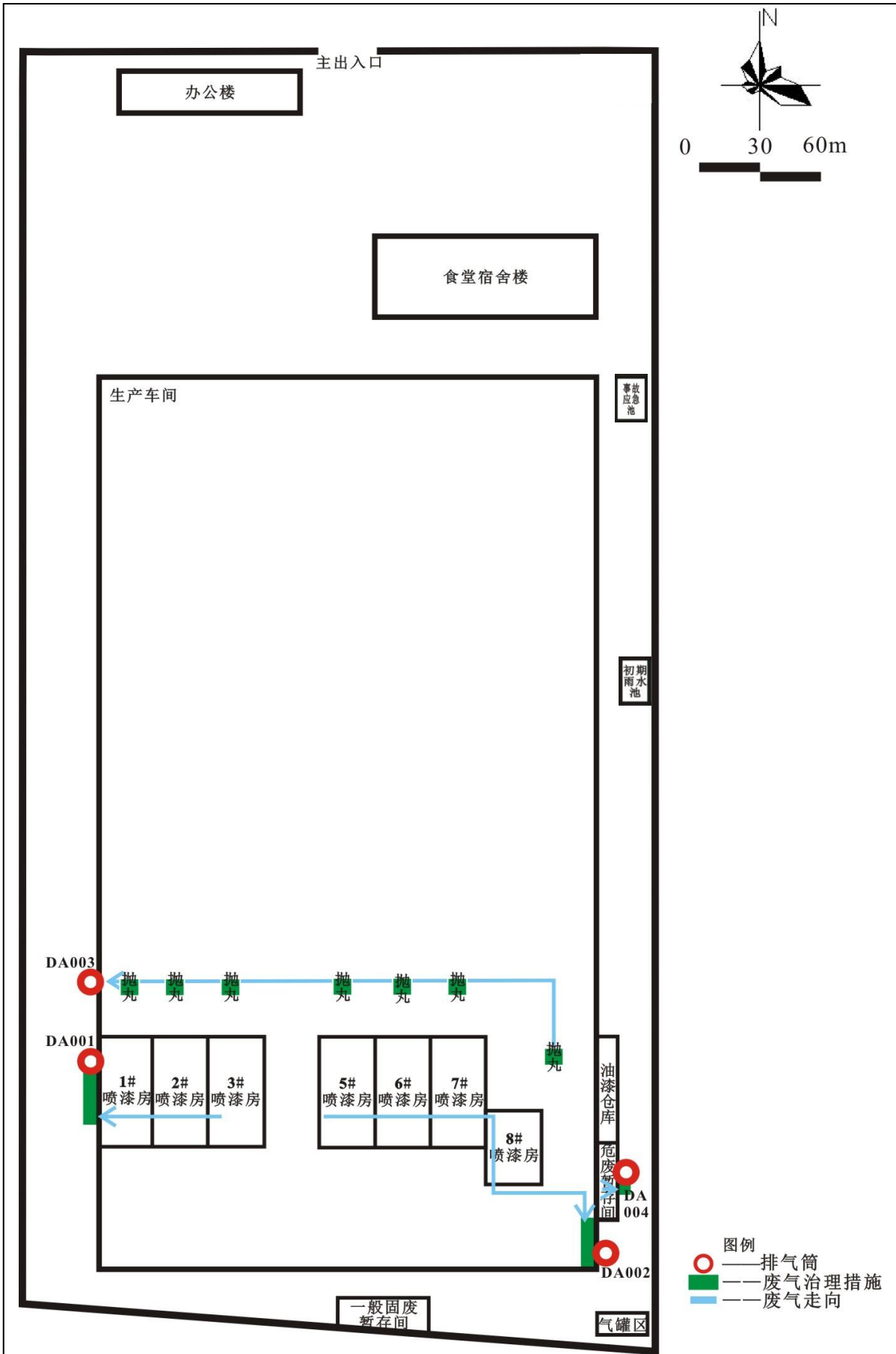
附图 4 项目废气走向图
