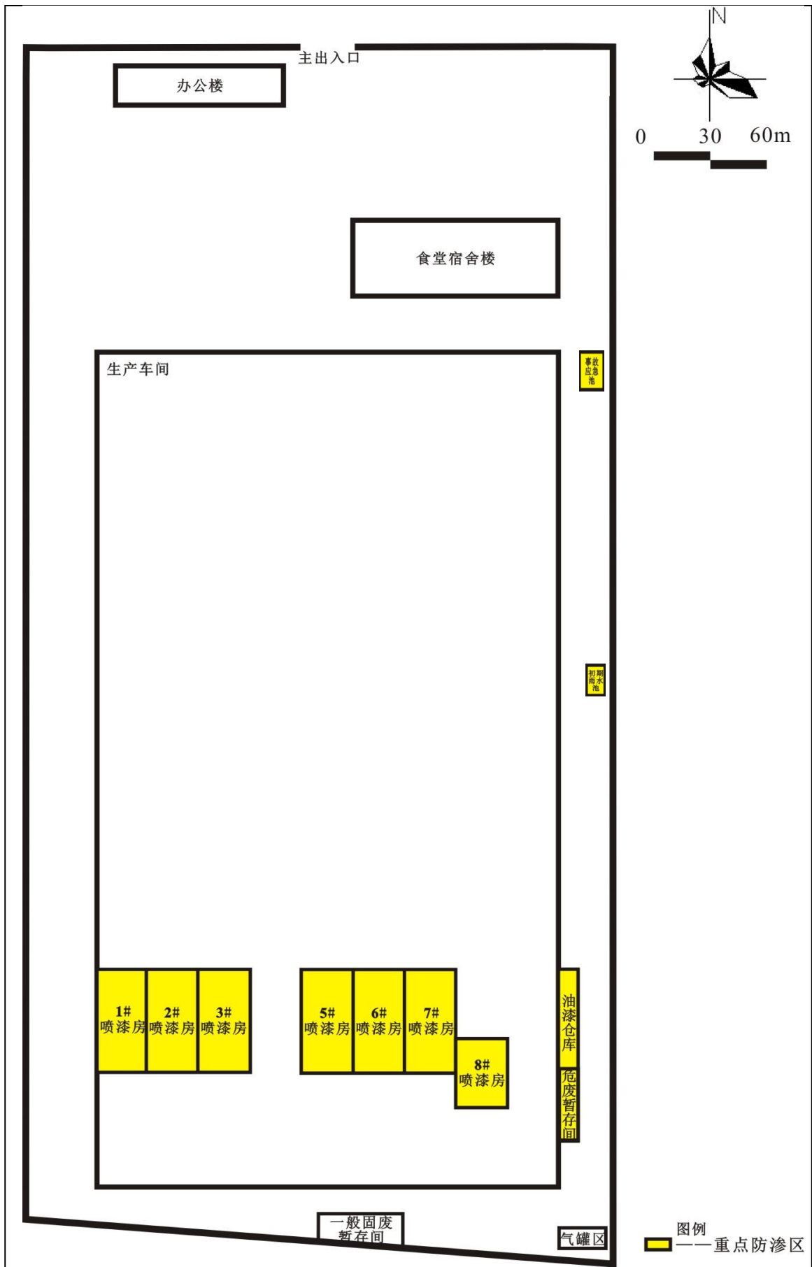
附图 6 项目分区防渗图
