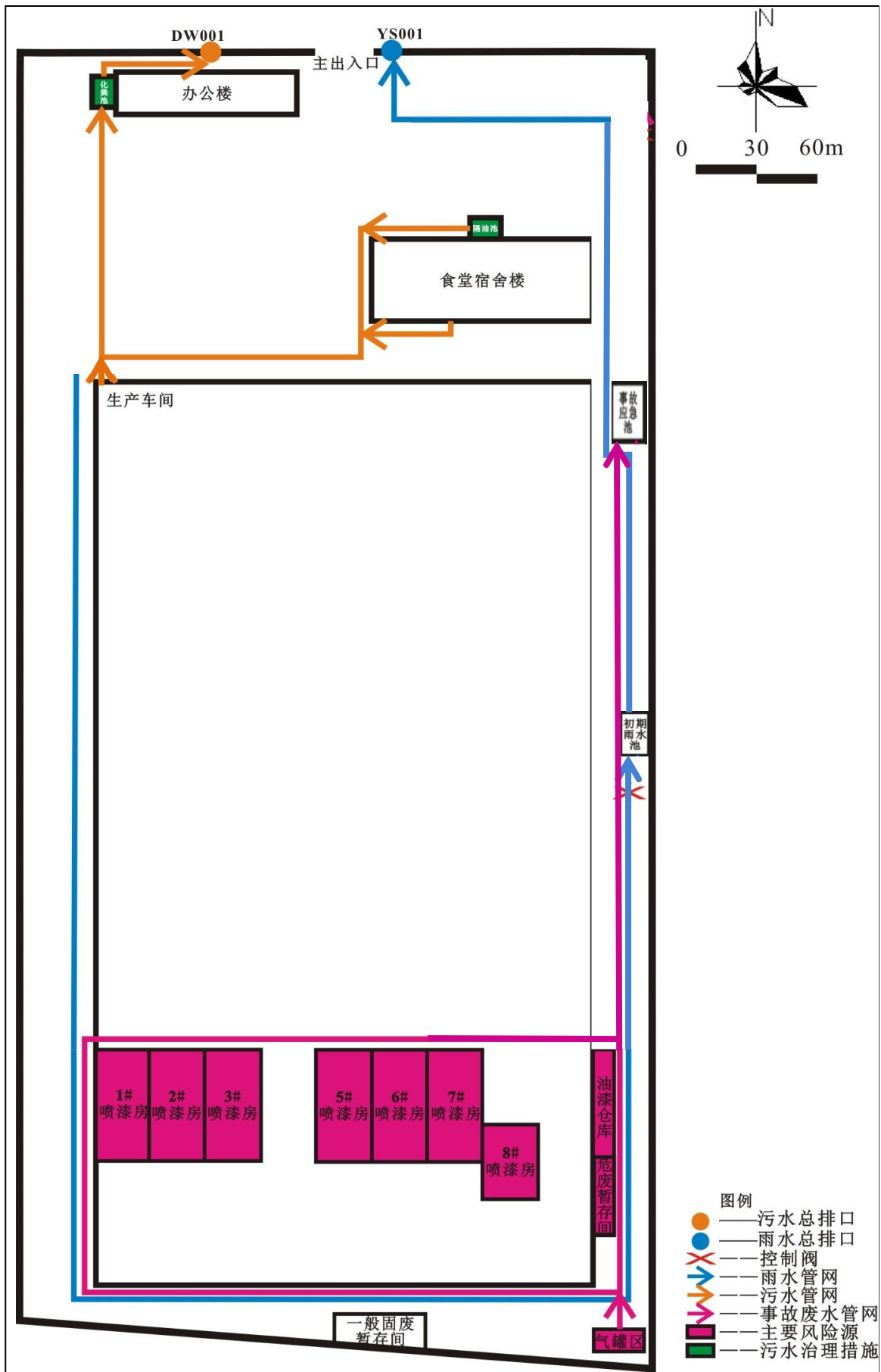
附图 5 项目雨污管网图
